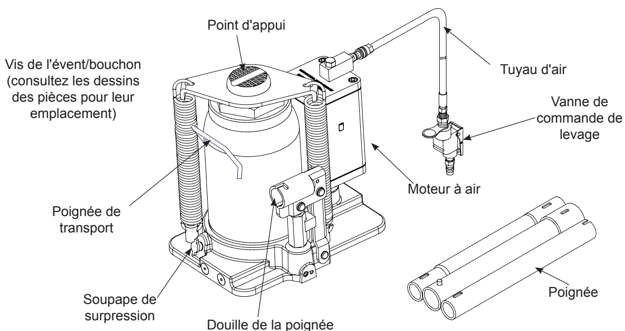
Figure 1 : Pièces des modèles 18126C et 18206C
