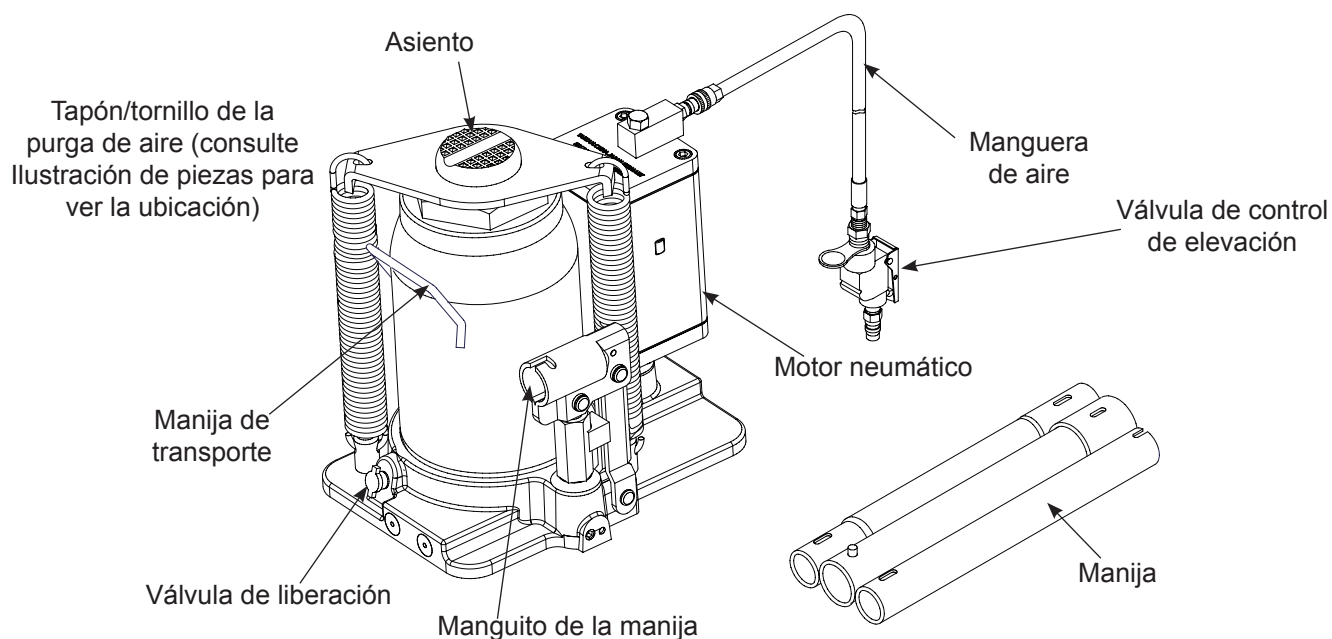
Figura 1: Nomenclatura de 18126C & 18206C
